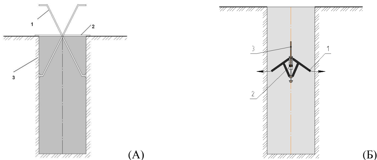
Рис. 1 Схемы измерения диаметра колонны.
